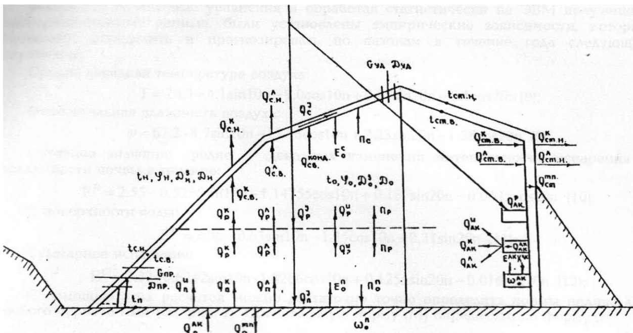
Рис. 2. Схема расчета тепло - и массообмена в солнечной теплице [5].
