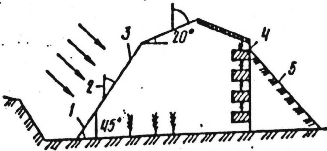
Рис.1 Гелиотеплица с автономным энергообеспечением: 1- опреснитель; 2- форточки для проветривания; 3 –остекление; 4-полки для рассады он также является аккумулятором тепла; 5 – с тыльно стороны грунтовая насыпь.
