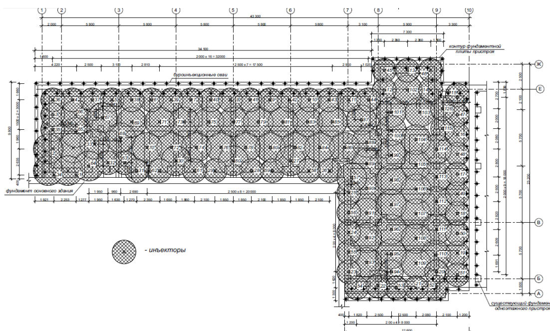
Рисунок 3. Схема уплотнения грунтового основания
