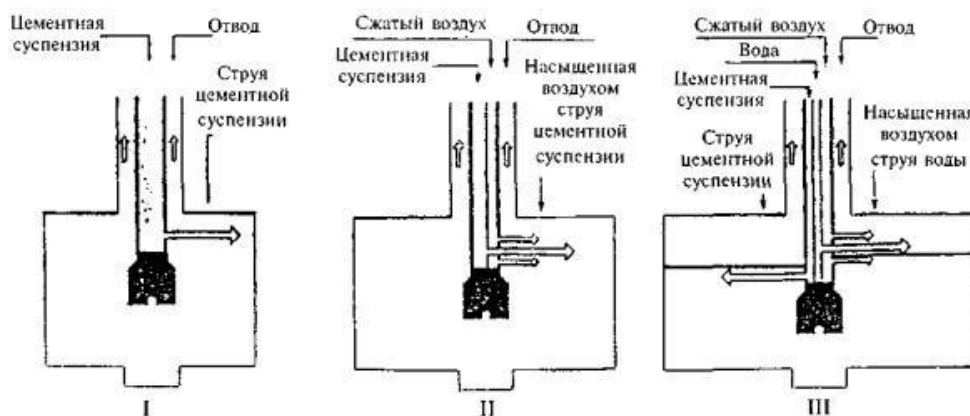
Рисунок 2. Варианты технологических режимов устройства грунтоцементных свай и массивов. I - однокомпонентная; II - двух- и III - трехкомпонентная технологии образования грунтоцемента.
