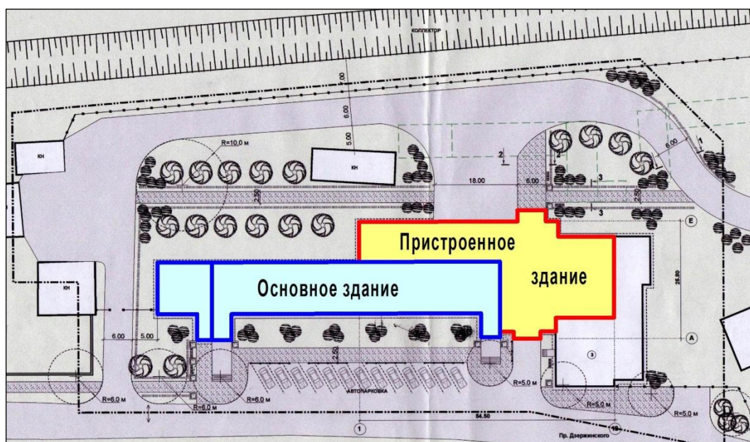
Рисунок 1. Ситуационный план застройки с торговым центром «Домострой»
